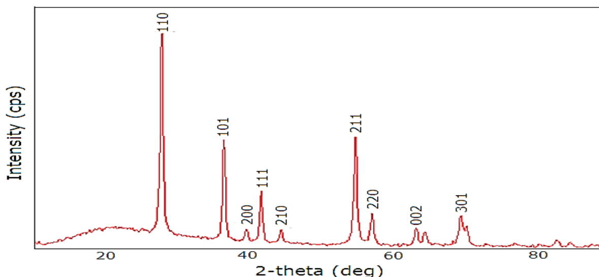
Şəkil 2. TiO 2 nanohissəciklərinin rentgen quruluşu (XRD)
