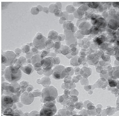
Şəkil 1. TiO 2 nanohissəcikləri üçün TEM görünüşü
